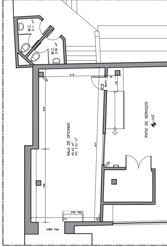
Planta Baixa - Sala de Oficinas Esc.: 1:100
