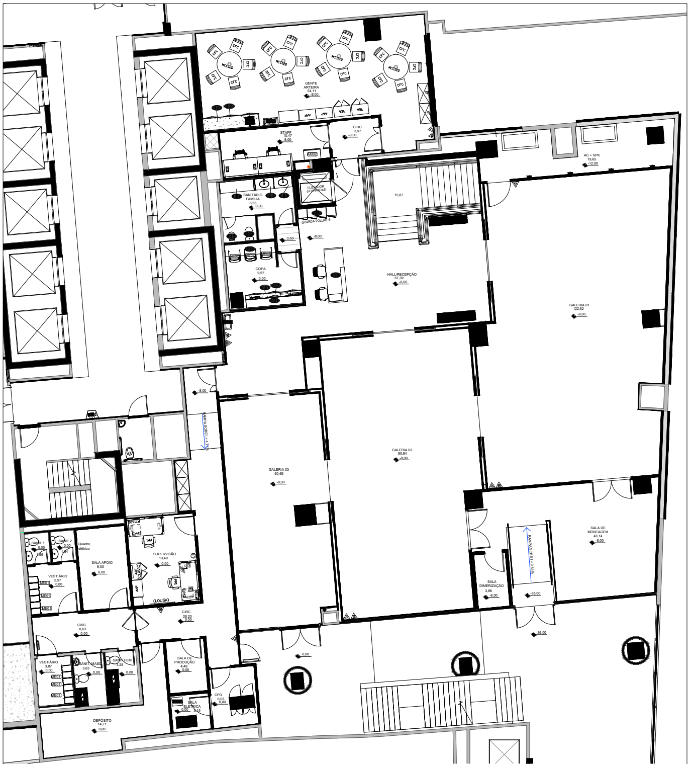
01 PL. BAIXA – 02º PAVTO (TORRE 2) Escala: 1/100
